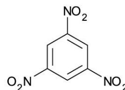
1. 1,3,5-Trinitrobenzene
