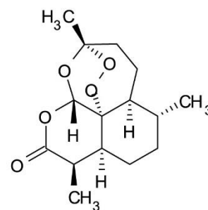
1. Artemisinin
