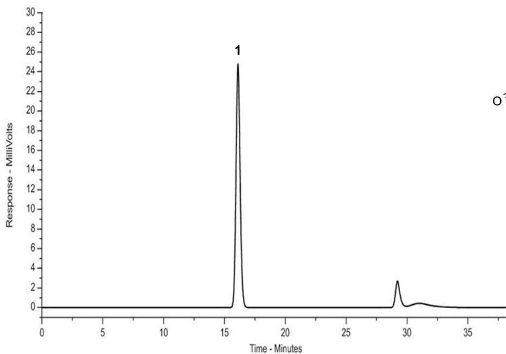
1. Artemisinin
