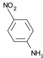
1. p-Nitroaniline
