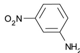
2. m-Nitroaniline
