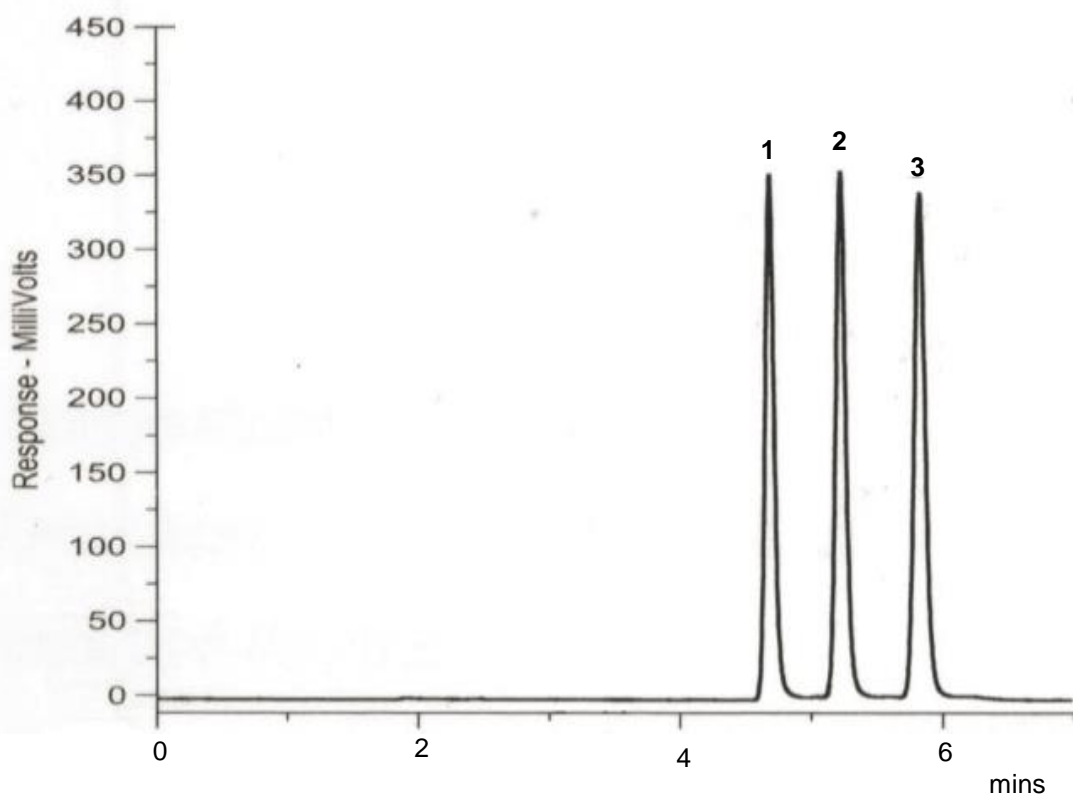
2. m-Nitroaniline
