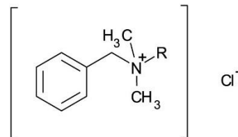
2. Benzalkonium chloride
