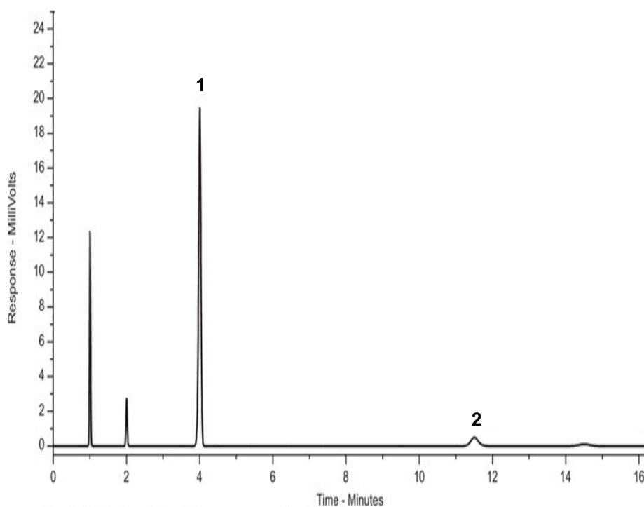
2. Benzalkonium chloride
