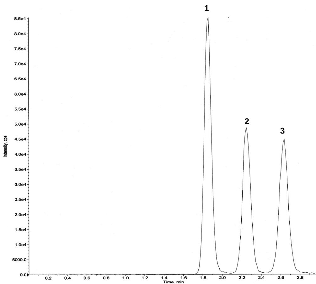
1. 6-epi-Pravastatin (MW: 424)
