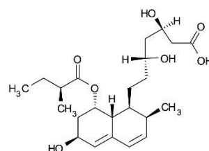
2. Pravastatin (MW: 424)
