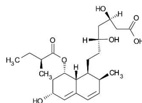
1. 6-epi-Pravastatin (MW: 424)
