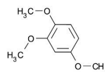
3. 1,2,4-Trimethoxybenzene
