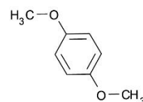
4. 1,4-Dimethoxybenzene
