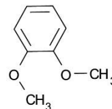
2. 1,2-Dimethoxybenzene
