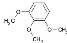
1. 1,2,3-Trimethoxybenzene
